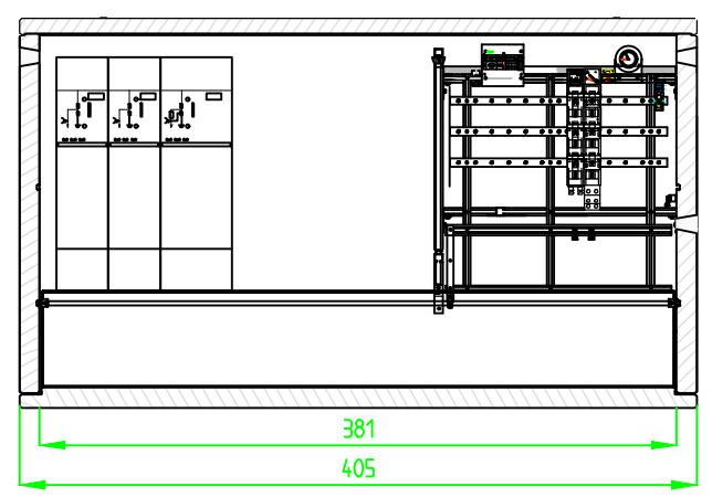
Coupe C-C
